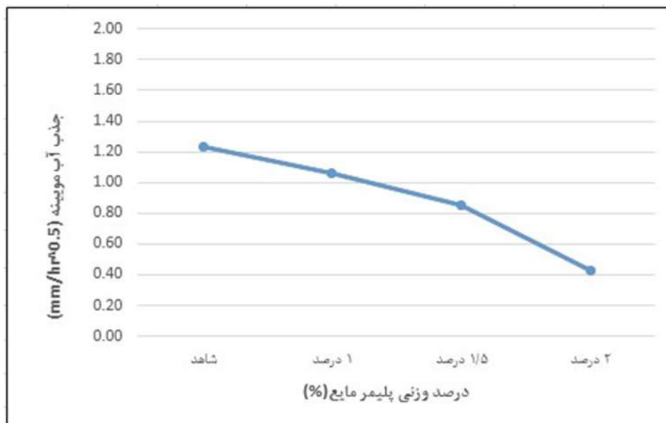
شکل شماره (۵) نمودار ضرایب جذب مویینگی آب در نمونه‌های ۷ روزه دارای پلیمر مایع
