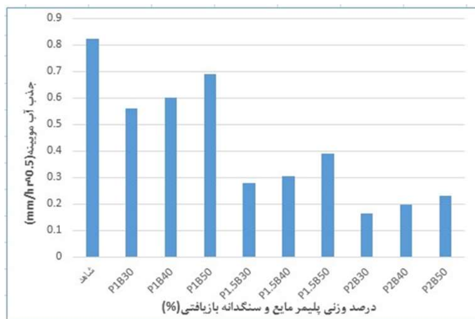
شکل شماره (۸) نمودار ضرایب جذب مویبندی آب در نمونه‌های ۲۸ روزه دارای پلیمر مایع و سنگدانه بازیافتی
