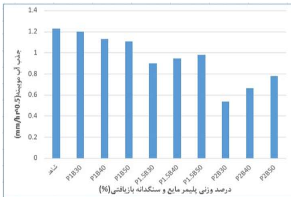
شکل شماره (۷) نمودار ضرایب جذب مویبگی آب در نمونه‌های ۷ روزه دارای پلیمر مایع و سنگدانه بازیافتی
