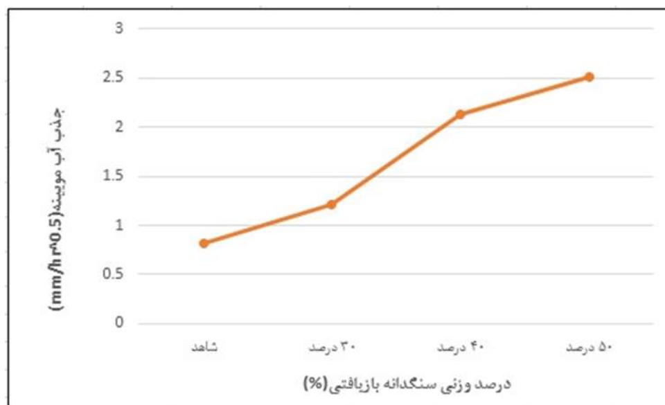
شکل شماره (۴) نمودار ضرایب جذب مویبگی آب در نمونه‌های ۲۸ روزه دارای سنگدانه بازیافتی
