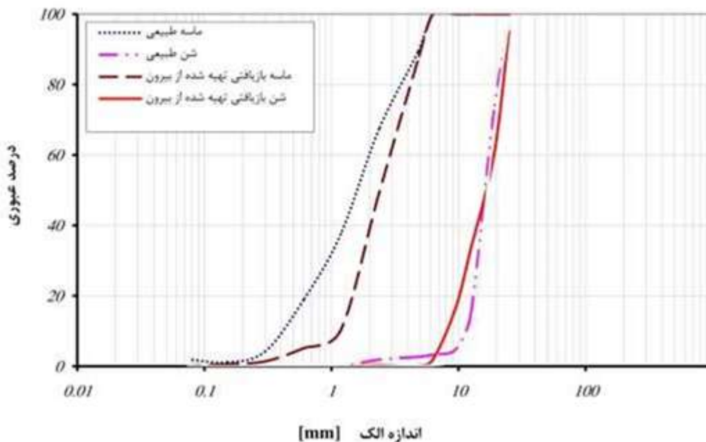
شکل شماره (۱): منحنی‌های دانه بندی مصالح سنگی
