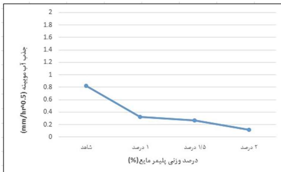
شکل شماره (۶) نمودار ضرایب جذب مویبگی آب در نمونه‌های ۲۸ روزه دارای پلیمر مایع
