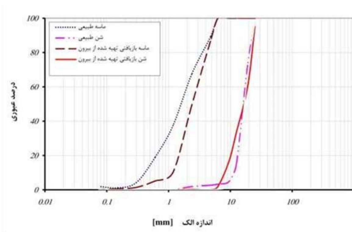
شکل شماره (۱): منحنی های دانه بندی مصالح سنگی
