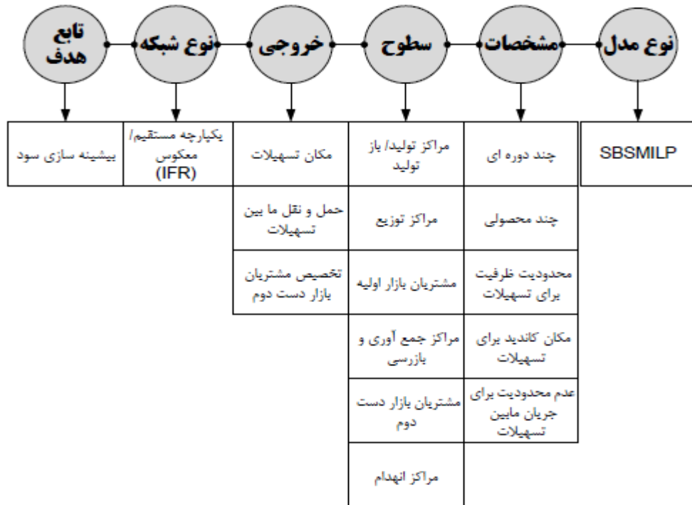
شکل (۲): ساختار شبکه پیشنهادی
