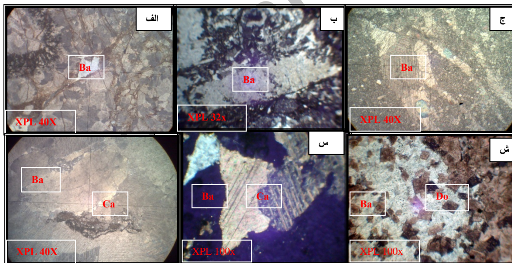
شکل ۲- الف) آغشتگی اکسید آهن در کنتاکت بین ماده معدنی و سنگ میزبان، ب) نمایی از یک بلور باریت نسل اول، ج) باریت در مسیر شکستگی ها و درز و شکافها مشاهده می شود (باریت نسل دوم)، د) نسل اول کانی کلسیت، س) بلورهای کلسیت در داخل رگه ها (نسل دوم کانی کلسیت)، ش) بلورهای لوزی شکل دولومیت بصورت انکلوزیون بر روی باریت تشکیل شده (نسل دوم کانی دولومیت)
