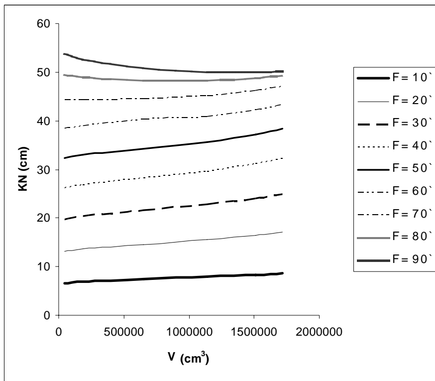
شکل ۴: منحنی KN-F در حالت بدون تریب
