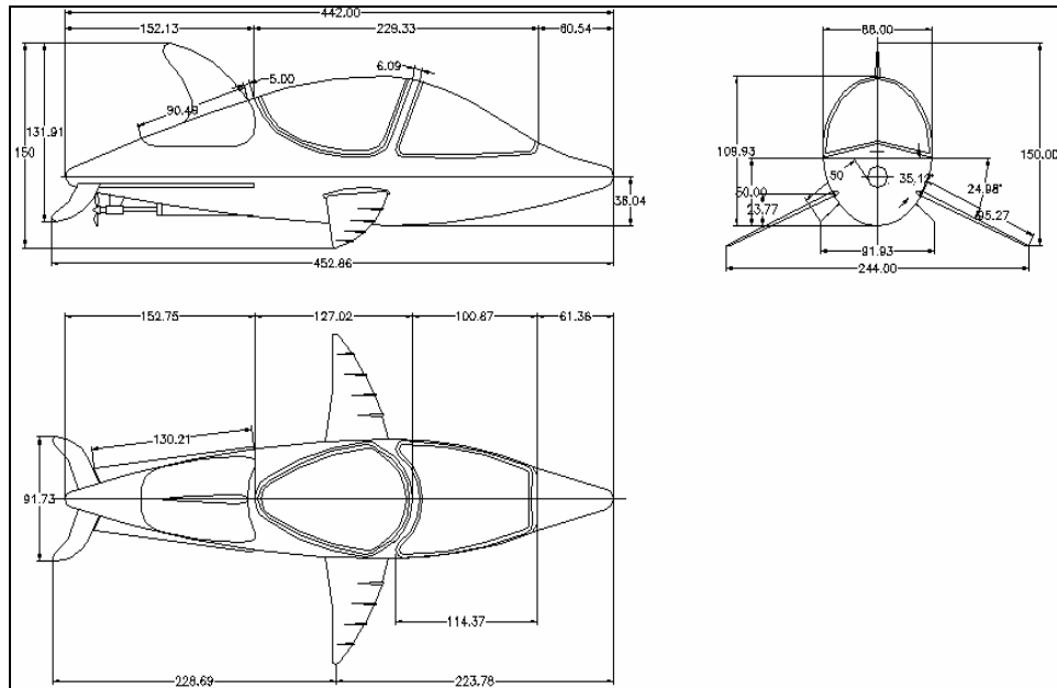
شکل ۲: جانمایی شناور
