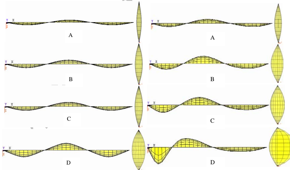
شکل ۱۱ تغییرات در مود تغییر شکل برای ورق نازک با نسبت ابعادی ۳ تحت اثر فشار محوری (راست: مود زین اسبی تغییر شکل اولیه، چپ: مود کمانشی تغییر شکل اولیه)
