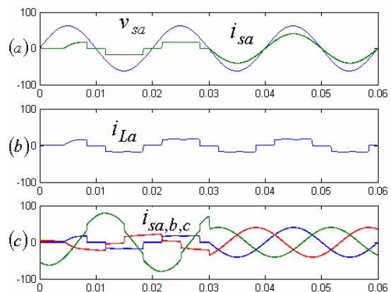
شکل ۹: (a) ولتاژ فاز a (ولت) و جریان طرف منبع فاز a (آمپر) (b) جریان بار فاز a (آمپر) (c) جریانهای سه فاز طرف منبع (آمپر)
