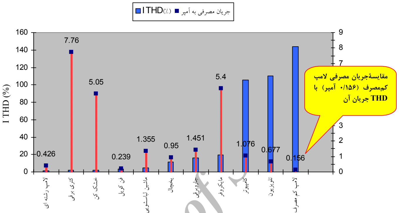
نمودار ۱- مقایسه جریان مصرفی و مقدار THD جریان هر مصرف کننده به تنهایی
