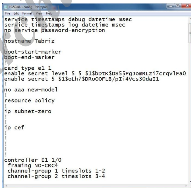
شکل ۴ پیکربندی روتر
