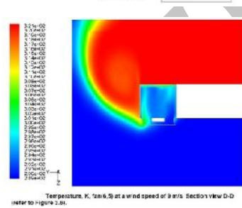
شکل ۷: ترموگرافی گردش ستون هوای داغ خروجی
