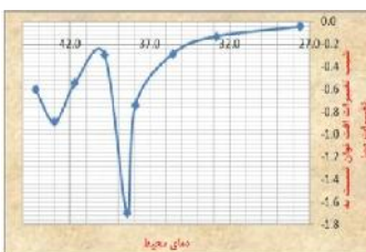
شکل ۳: شیب تغییرات افت توان نسبت به تغییرات دمای محیط
