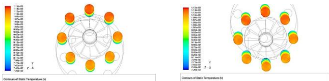
د- زاویه پره‌های هادی ۶۰ درجه- مسیر هوای ثالثیه باز نمای از بالا نمای از پایین
