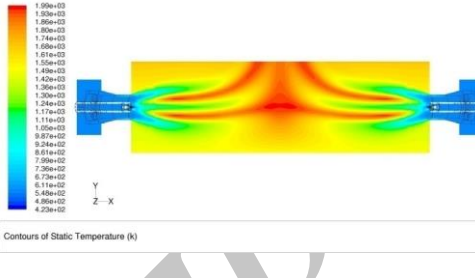
ب- زاویه پره‌های هادی ۴۵ درجه- مسیر هوای ثالثیه باز
