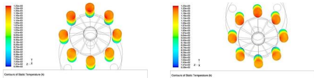
ج- زاویه پره‌های هادی ۴۵ درجه- مسیر هوای ثالثیه بسته نمای از بالا نمای از پایین
