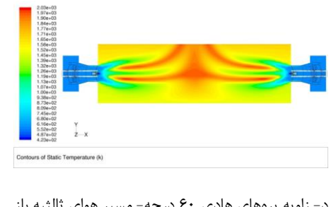
د- زاویه پره‌های هادی ۶۰ درجه- مسیر هوای ثالثیه باز
