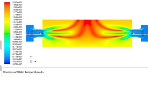
ج- زاویه پره‌های هادی ۴۵ درجه- مسیر هوای ثالثیه بسته
