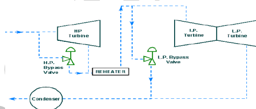
(شکل 1) موقعیت کنترل ولو HP BY PASS در سیکل
