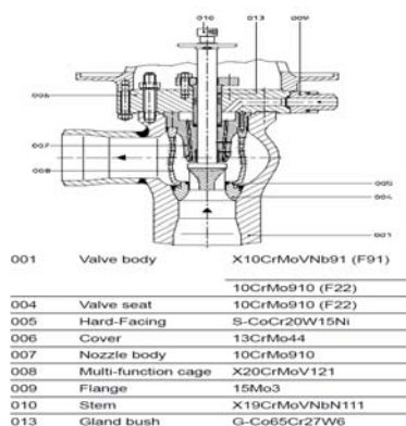
(شکل 7) - جنس قسمتهای مختلف والو
