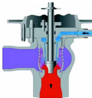
( شکل 4) بخار با دمای 537 درجه و فشار 167 بار
