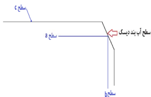
(شکل 10) سطوح مورد بررسی در آزمون سختی سنجی.
