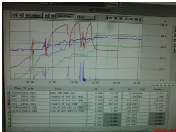
(شکل 3)- نوسانات ایجاد شده در هنگام نشستی داخلی والو
