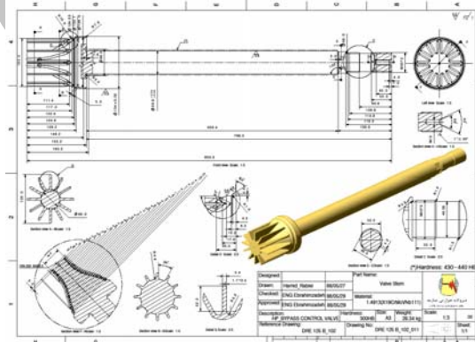
(شکل شماره 6) - نقشه استم والو
