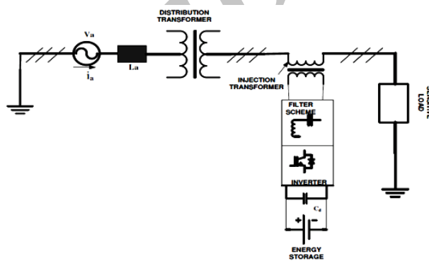
شکل ۱: بلوک دیاگرام کلی بازیاب دینامیکی ولتاژ [۱۹].
