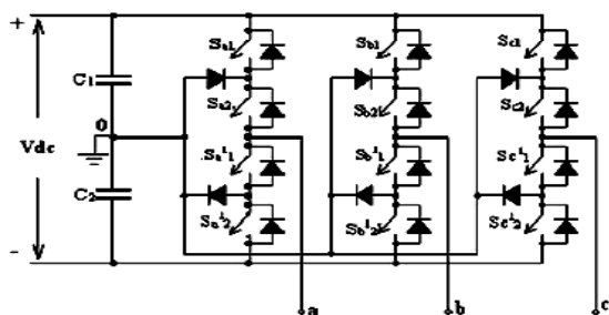
شکل ۳: مبدل سه فاز سه سطح دیود کلمپ [۲۰].
