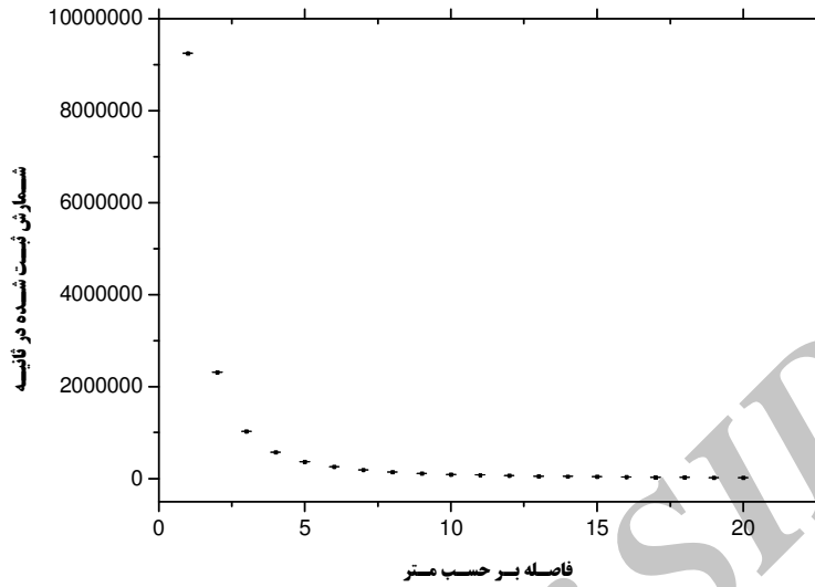
شکل شماره ۳- نتایج حاصل از شبیه سازی تعداد ذره وارد شده از چشمه ۱۰۰ میلی کوری به آشکارساز در فاصله ۱ تا ۲۰ متری، با استفاده از تالی استار اف ۸ کد MCNP4c
