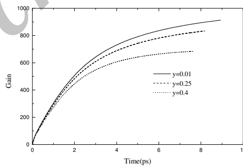
شکل ۳: مقایسه بهره در قرص سوخت D / T_{x=0.01} / {}^3\text{He}_y به ازای نسبت های مختلف ناخالصی هلیوم-۳
