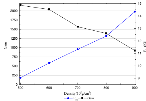
شکل ۱: مقادیر عددی بدست آمده بهره انرژی در قرص سوخت D / T_{x=0.01} / {}^3\text{He}_y y=0.18
