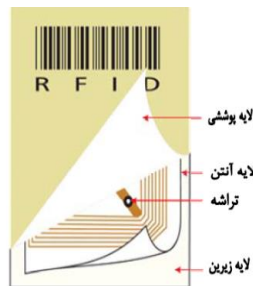
شکل ۴ - تگ RFID در قالب کارت
