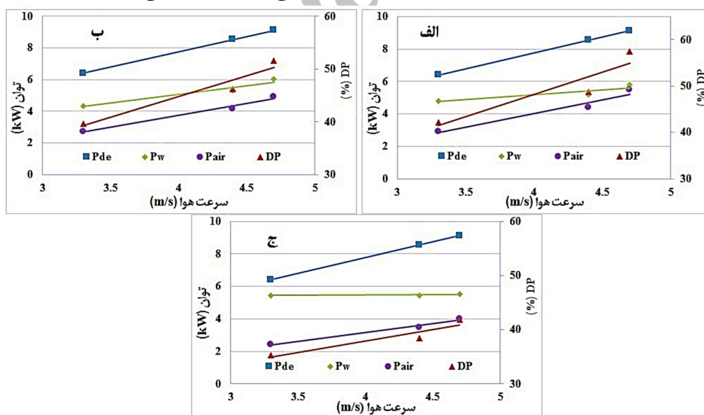
شکل ۸- تغییرات توان سرمایشی مورد نیاز P_{de} ، توان از دست داده توسط هوا P_{air} ، توان جذب شده با آب P_a ، و درصد کاهش توان مورد نیاز (DP) در سرعت های مختلف و دبی های، الف) ۱۳ lit/min، ب) ۱۱/۵ lit/min و ج) ۱۰ lit/min
