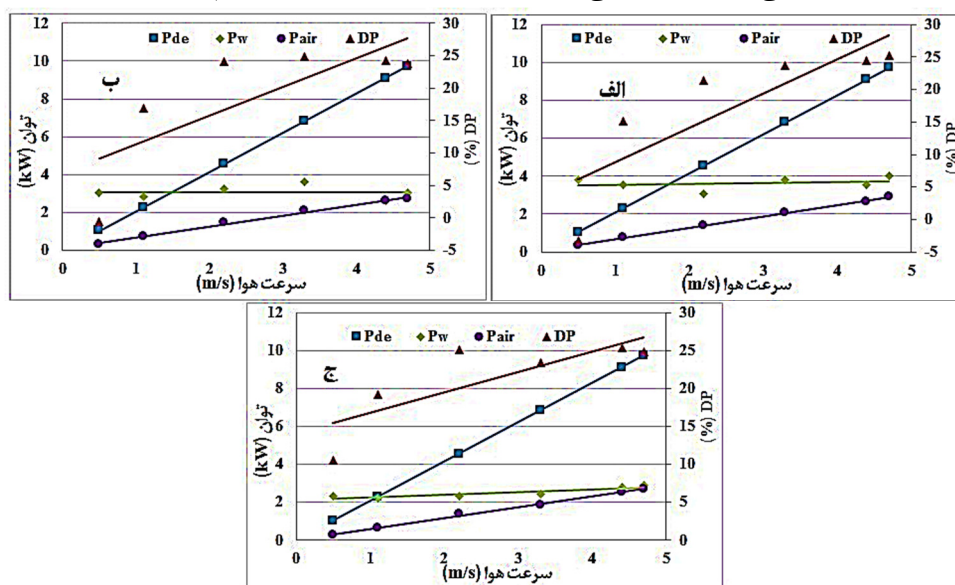
شکل ۴- تغییرات توان مورد نیاز ( P_{de} )، درصد کاهش توان مورد نیاز (DP)، توان دریافتی هوا ( P_{air} ) و توان از دست داده شده آب ( P_w ) در سرعت های مختلف (الف) دبی ۳۴ lit/min - (ب) دبی ۲۹ lit/min و (ج) دبی ۱۶ lit/min
