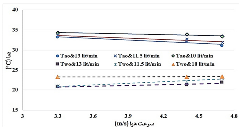
شکل ۷- تغییرات دمای هوا و آب در طول فرایند سرمایش
