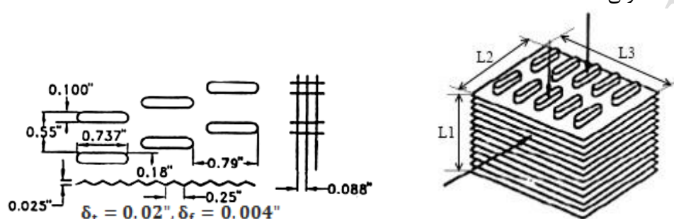
شکل ۱: مشخصات هندسی مبدل SR-۷۳۷-۰/۱۱/۳۲ [۲].
