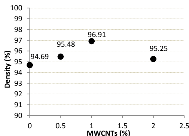
شکل ۱۰- نمودار چگالی نسبی کامپوزیت‌های آلومینیوم ۷۰۶۸- نانولوله‌های کربنی با قطر متوسط ۶۵ نانومتر.
