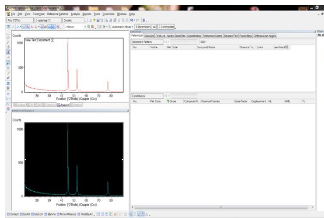
شکل ۴- تحلیل منحنی‌های الگوی پراش اشعه ایکس برای پودر آلومینیوم ۷۰۶۸ توسط نرم افزار xpert high score.
