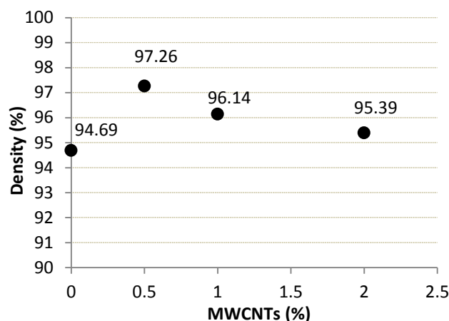
شکل ۹- نمودار چگالی نسبی کامپوزیت‌های آلومینیوم ۷۰۶۸- نانولوله‌های کربنی با قطر متوسط ۱۰ نانومتر.
