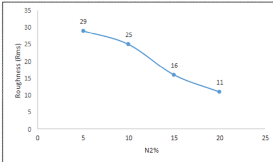
شکل 3: تغییرات زبری سطح در غلظت‌های مختلف نیتروژن.
