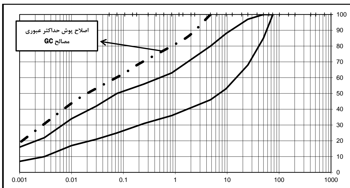
شکل ۱- اصلاح پوش حداکثر عبوری مصالح GC
