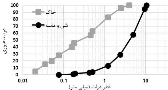
شکل (۲): منحنی دانه‌بندی پوشش معدنی و خاک
