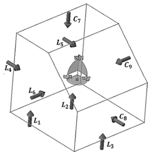
شکل ۱۴ قطعه کار با سیستم جاسازی و بست مشخص شده(حالت ۱)
