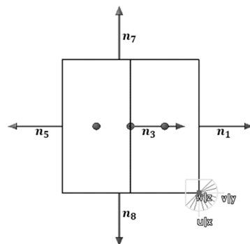
شکل ۶ تصویر قطعه کار در صفحه xy
