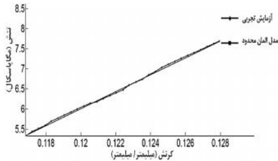
شکل ۸. نمودار تنش کرنش برای اندازه مش ۰/۱۶ و آزمون تجربی
