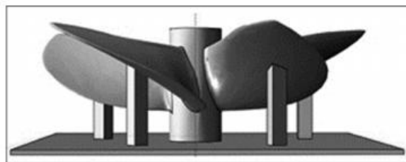
شکل ۲ فیکسچر مورد استفاده برای ماشین‌کاری پروانه
