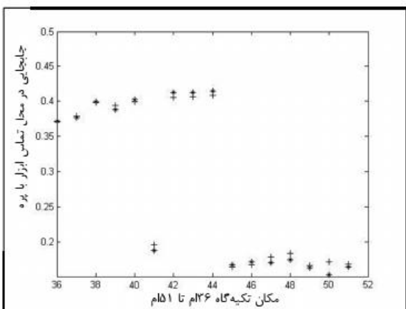
شکل ۱۱. کیفیت آموزش شبکه و میزان تطابق نتایج آن با نتایج به دست آمده توسط تحلیل اجزا محدود
