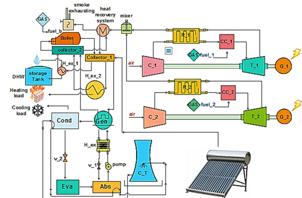
Fig.1 schematic of a solar assisted triple co-generation system شکل 1 شماتیک سیستم تولید سه گانه (CCHP) کمک خورشیدی
