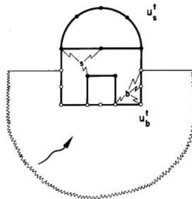
سیستم خاک و سازه
