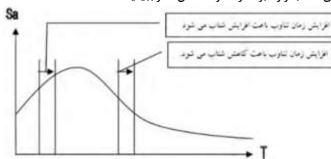
تغییرات شتاب نسبت به زمان تناوب
