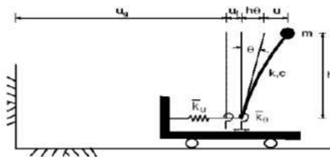
تغییر مکان جانبی سازه بر اثر حرکات افقی و گهواره ای پی
