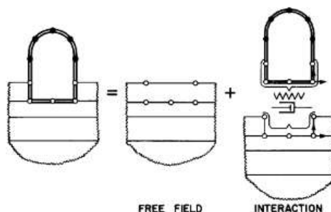
روش زیرسازه برای تحلیل اندرکنش خاک-سازه
