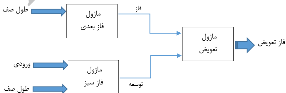
شکل ۲- دیاگرام شماتیک از کنترل کننده‌ی فازی سوگنو
