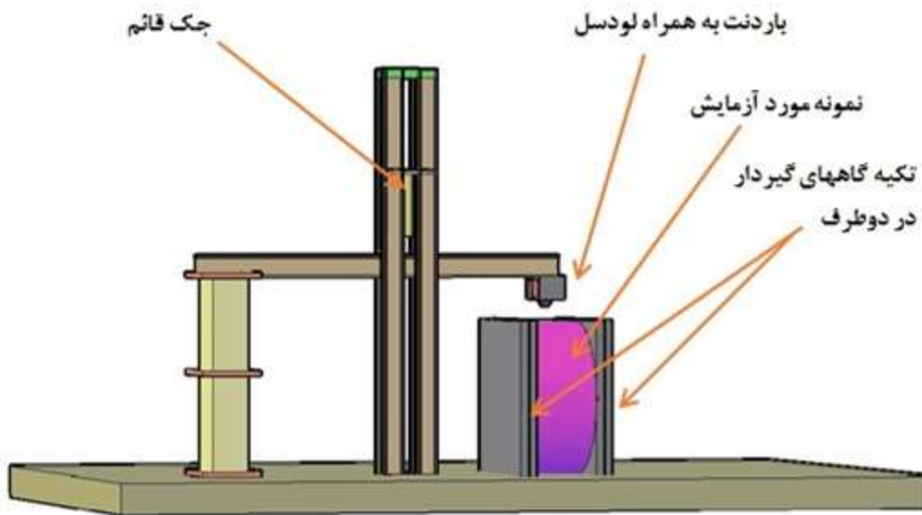
شکل ۴: شکل شماتیک نمونه در آزمایشگاه
