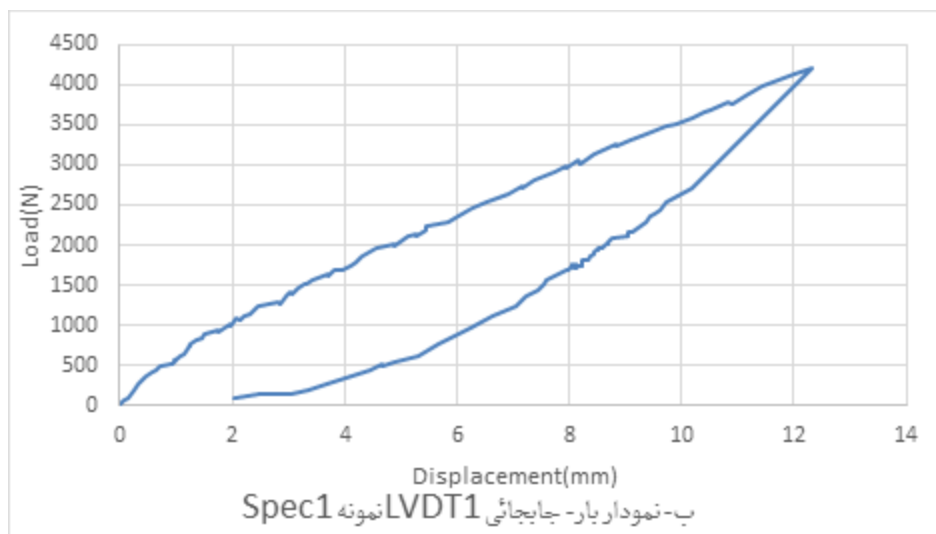
شکل ۸: نمودارهای بدست آمده از آزمایش اول
