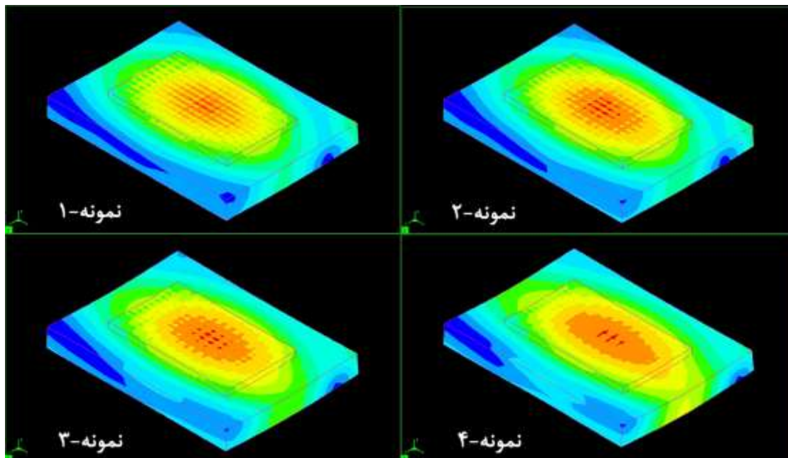
شکل ۴- نمایی توزیع اعوجاج در نمونه‌های مورد بررسی
