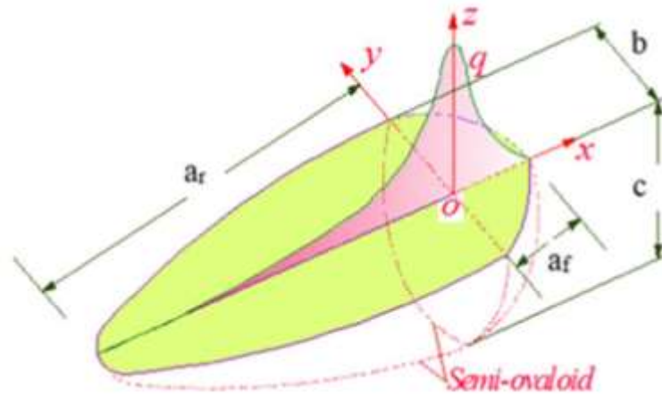
شکل ۳- مدل منبع حرارتی استفاده شده در تحلیل‌ها [۱۱]
